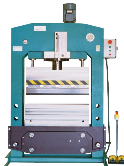
Presse de 200 to avec en option un équipement de pliage de 1020 mm
