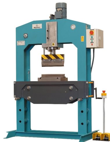
Presse de 80 to avec en option un équipement de pliage de 415 mm.
